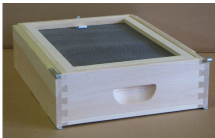
Abb.9: MS-Deckel-Futtertrog Darstellung mit Abdeckrahmen
